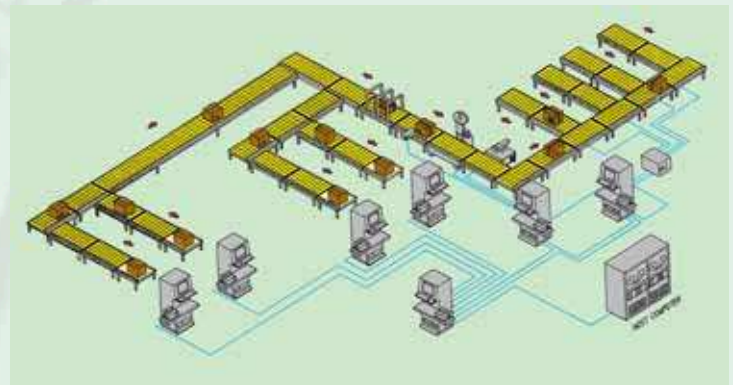
Linee per la preparazione degli ordini con interfacciamento in tempo reale al sistema gestionale aziendale. Lines for order execution with host computer interface in real time.
